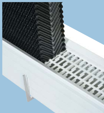
Zásobník pro vodu s pevnou nosnou konstrukcí pro 2H HUMIPACKING® výplně
