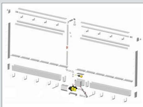
Systém 2H AGRIdek je sestaven za pomoci spojů, které lze jednoduše zacvaknout do sebe, v konečné fázi montáže jsou díly lepené.
